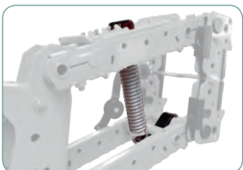
Zusatzkit Säaggregat Belastungsfeder.
